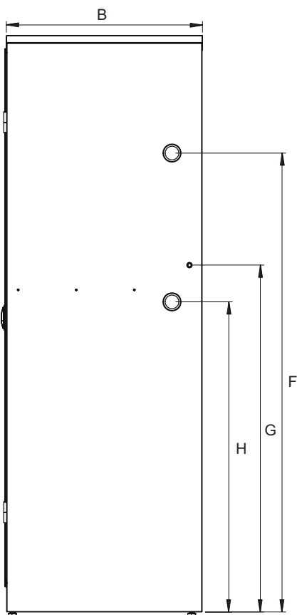
Seitenansicht rechts
