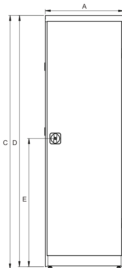
Frontansicht
